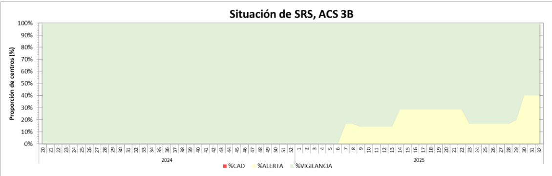
Figura N° 2. Proporción de centros según categoría, PSEVC-Piscirickettsiosis, ACS 3B. (Fuente: Sernapesca).
