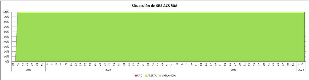
Figura N° 2. Proporción de centros según categoría, PSEVC–Piscirickettsiosis, ACS 50A. (Fuente: Sernapesca).
